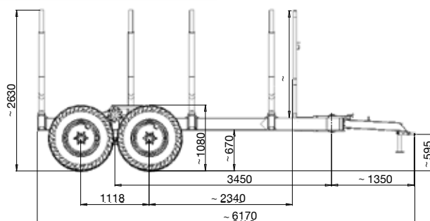
Dimensions avec roues en option
