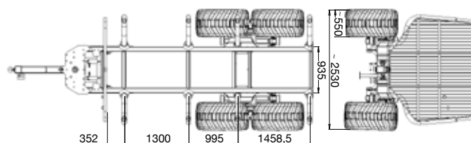
Dimensions avec roues en option
